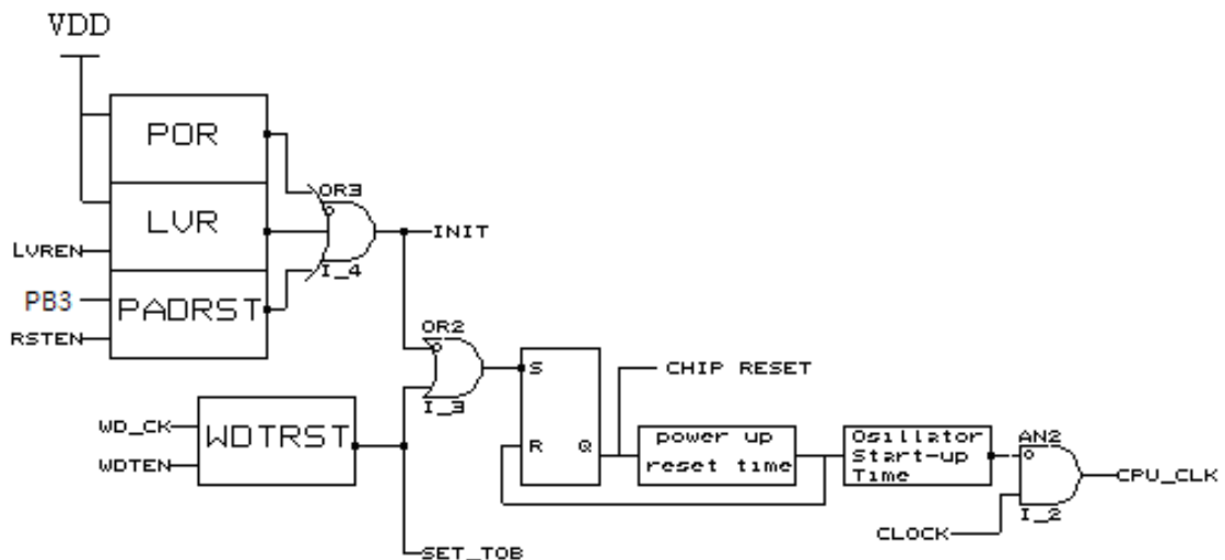
图 25 芯片复位电路框图
